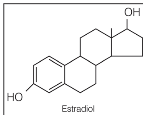
Figura 1. Molécula de estradiol, mostrando o anel fenólico e a posição 17 contendo uma hidroxila (OH). No 17 \beta -estradiol, este grupamento encontra-se em conformação \beta .
